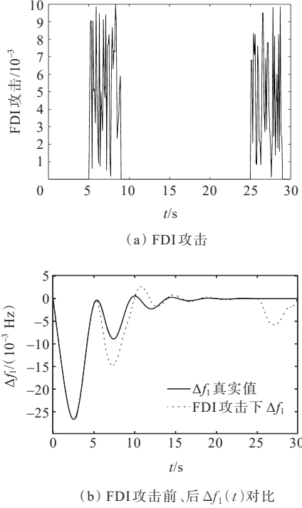
图6 FDI攻击下 \Delta f_1(t)
