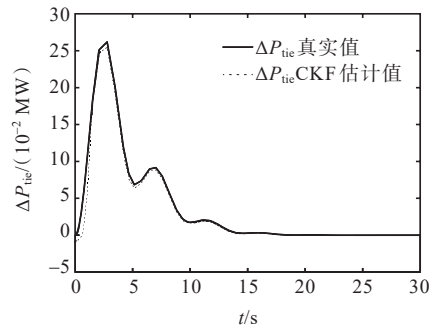
(c) 联络线的功率 \Delta P_{tie}(t)
