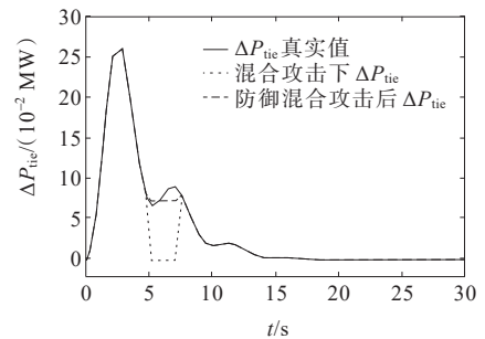
图8 混合攻击的防御
