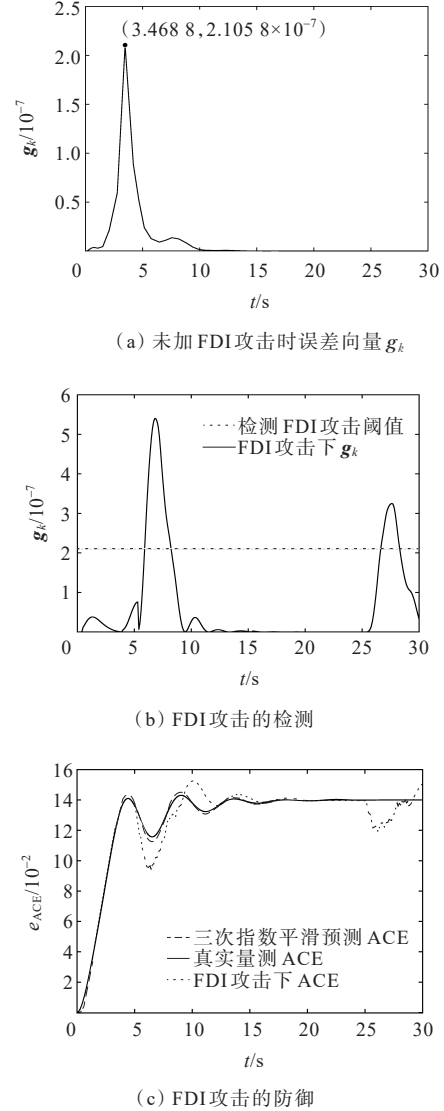
图7 FDI攻击的检测与防御
