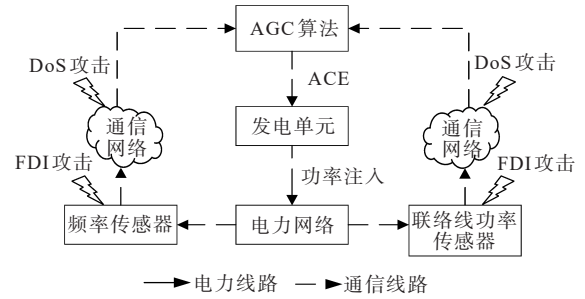
图2 存在潜在网络攻击的LFC系统框图
