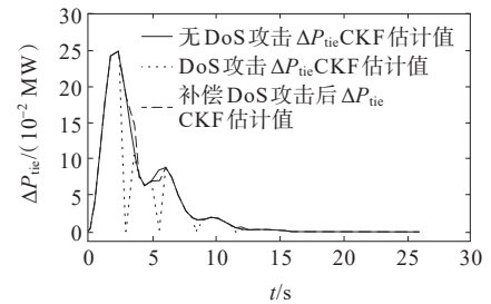
(c) 防御DoS攻击后CKF估计值
