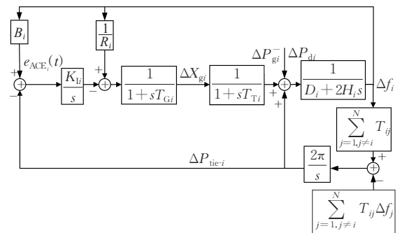
图1 多区域电力系统第 i 个区域的LFC框图
