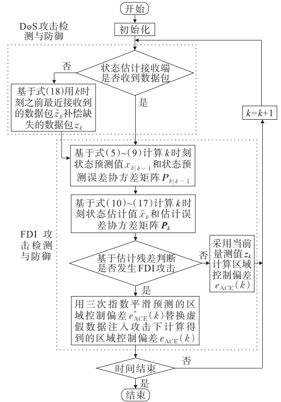
图3 混合攻击下基于CKF的多区域电力系统的检测与防御流程
