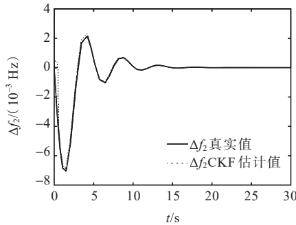
(b) 系统频率偏差 \Delta f_2(t)
