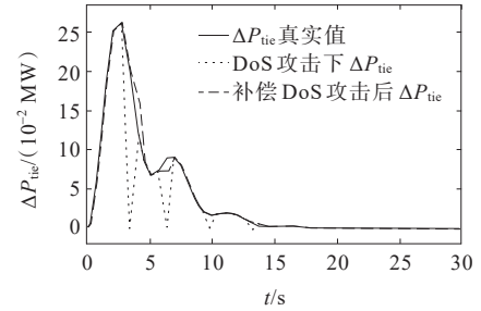
(b) DoS攻击的防御
