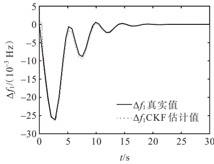
(a) 系统频率偏差 \Delta f_1(t)
