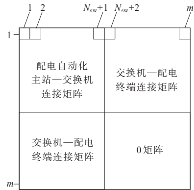
图4 配电网CPS信息层连接矩阵
