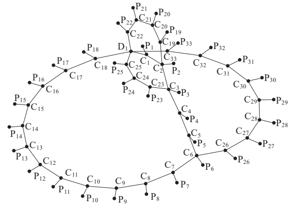
图10 传统拓扑方案的拓扑连接
