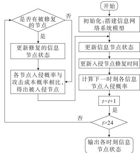
图3 配电网CPS蠕虫病毒传播模型框架
