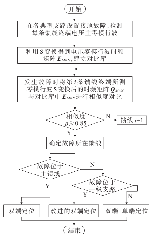
图5 故障选线和精确定位的流程
