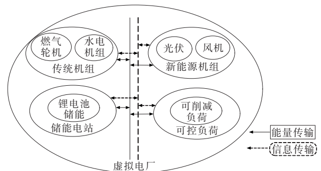
图1 虚拟电厂内部结构
