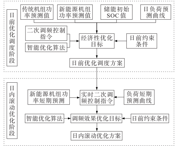
图2 VPP两阶段优化流程
