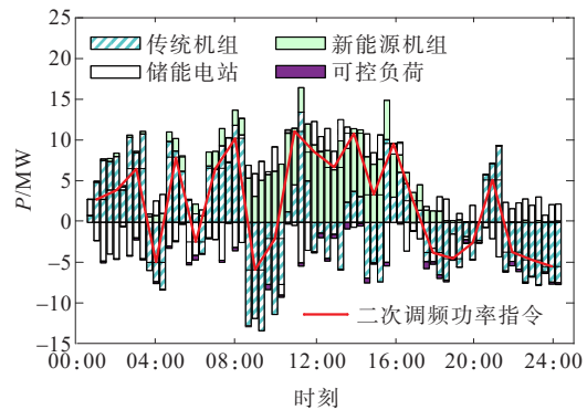
图 5 方案 1~3 各机组输出功率
