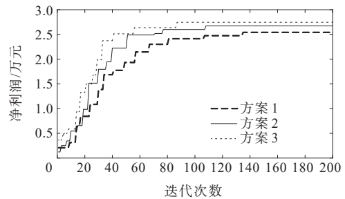
图 4 3 种方案下算法收敛情况对比
