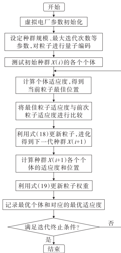
图3 改进的QPSO算法流程
