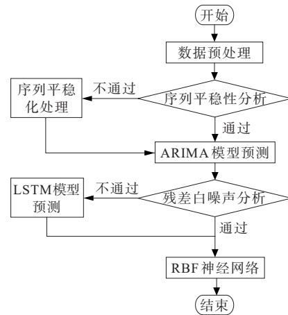
图6 组合模型流程
