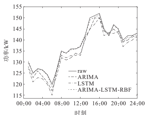
图9 3种模型的预测值对比(9月20日)
