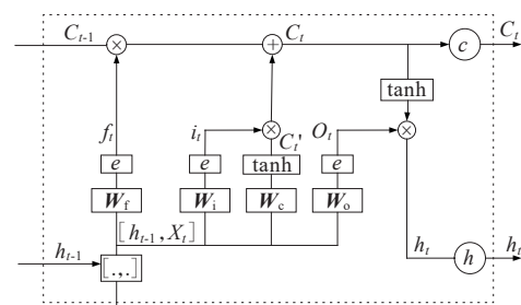
图4 LSTM模型
