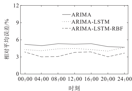
图10 风机出力预测误差对比
