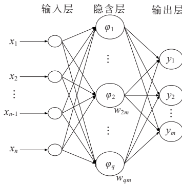
图5 RBF神经网络结构
