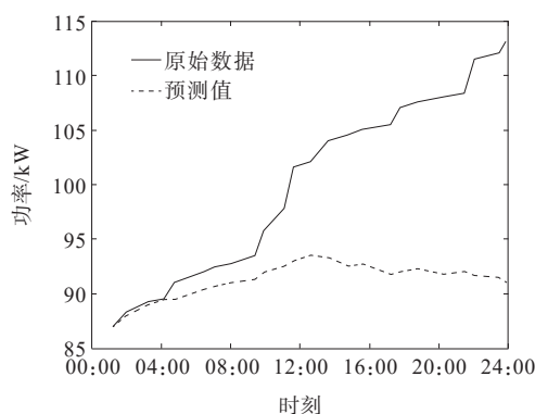
图7 原始值与预测值对比(7月27日)
