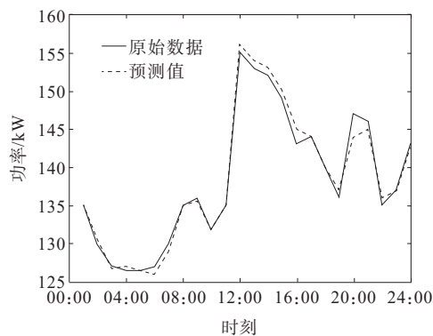
图8 原始值和预测值对比(8月26日)
