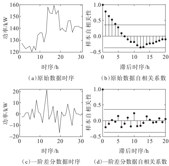
图3 平稳性分析
